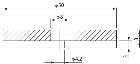
垫板·圆形·白φ50· 微型气缸用
