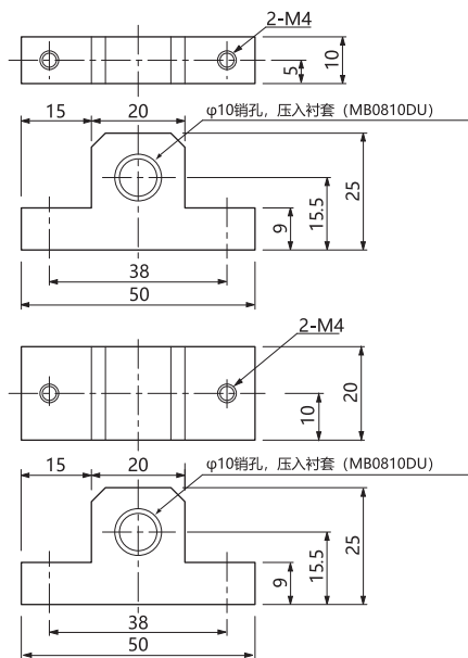
滑移板·微型气缸用
