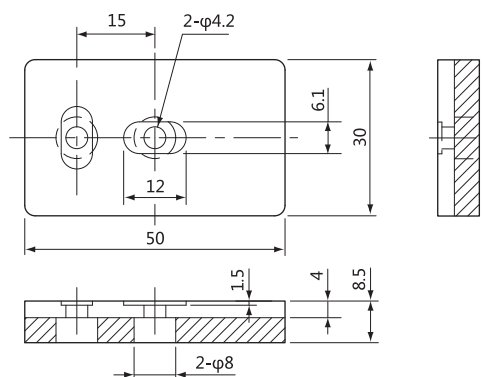
垫板·方形·白 2孔· 微型气缸用
