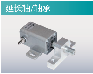
延长轴/轴承 延长微型气缸的导杆,用轴承固定轴的运动导向。
